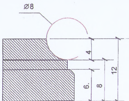
profil podstawy - kredensja
