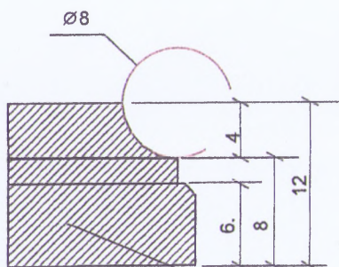
profil podstawy - ambona
