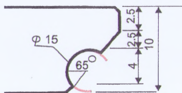
profil górnej płyty - kredensja
